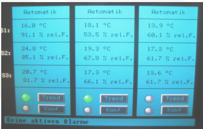
Einstellung und Anzeige der SOLL- und IST-Werte der Feuchtigkeit
